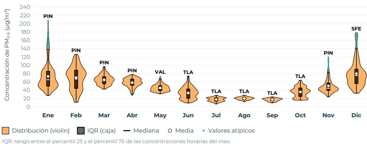
Figura 15. Distribución horaria mensual de PM 2.5 (promedio móvil de 24 horas) en el AMG, 2024.
