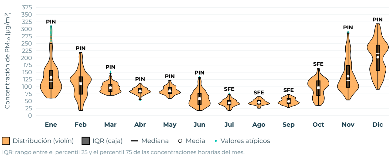
Figura 12. Distribución horaria mensual de PM 10 (promedio móvil de 24 horas) en el AMG, 2024.
